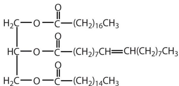
triglyceride - A
