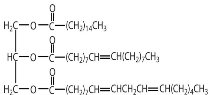
triglyceride - B
